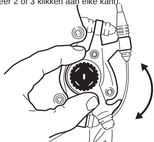
De afstelknop van het buitenste remblokje
